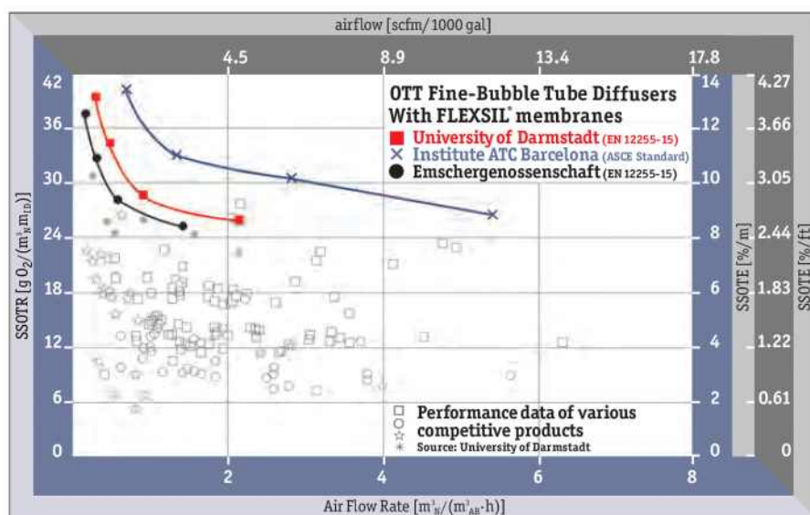
Membránové provzdušňovače od firmy OTT zajišťují jemnobublinnou aeraci.
