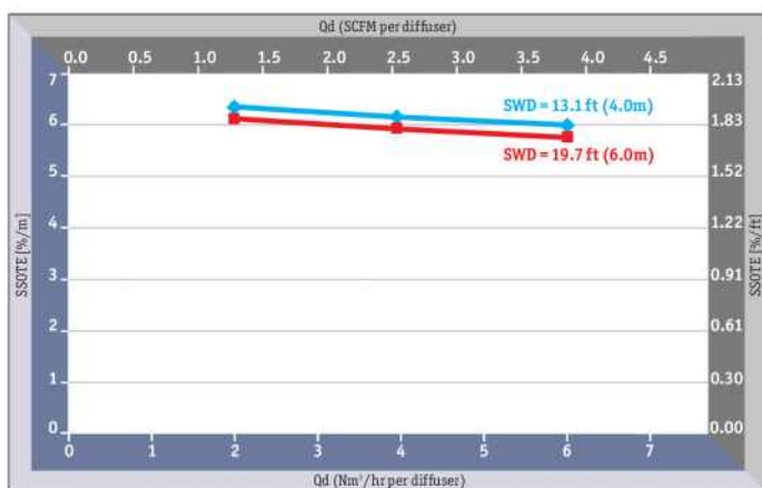
SSOTE a propustnost při hustotě osazení 1 D-REX® provzdušňovač na 1m 2
